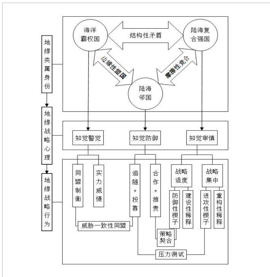
图 1 北极地缘政治行为体互动模型
